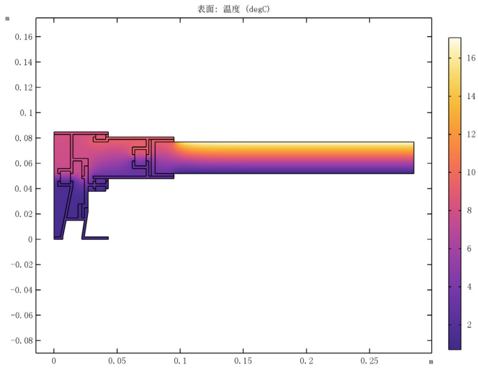
图 14: 推拉窗的温度分布。
