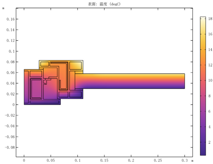
图12: 内含钢条的PVC 框架的温度分布
