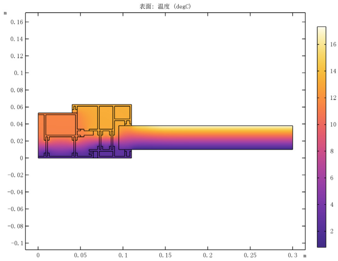
图10: 带隔热层的铝质框架的温度分布。
