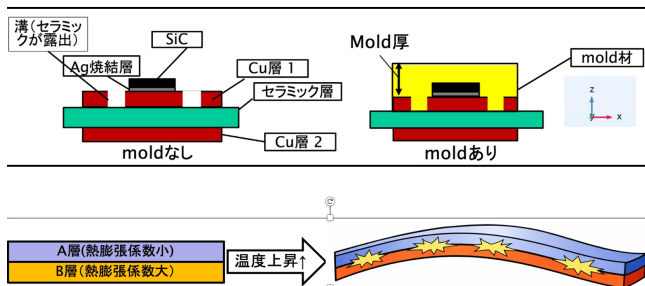
図1. 上: SiCチップ搭載AMB基板の断面図.
