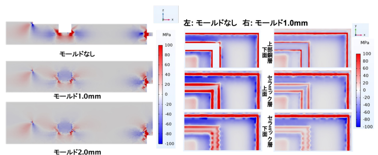
図2. 左: 垂直方向垂直応力の垂直方向断面図 (変形なし). 右: 垂直方向垂直応力の水平方向断面図 (変形なし).
